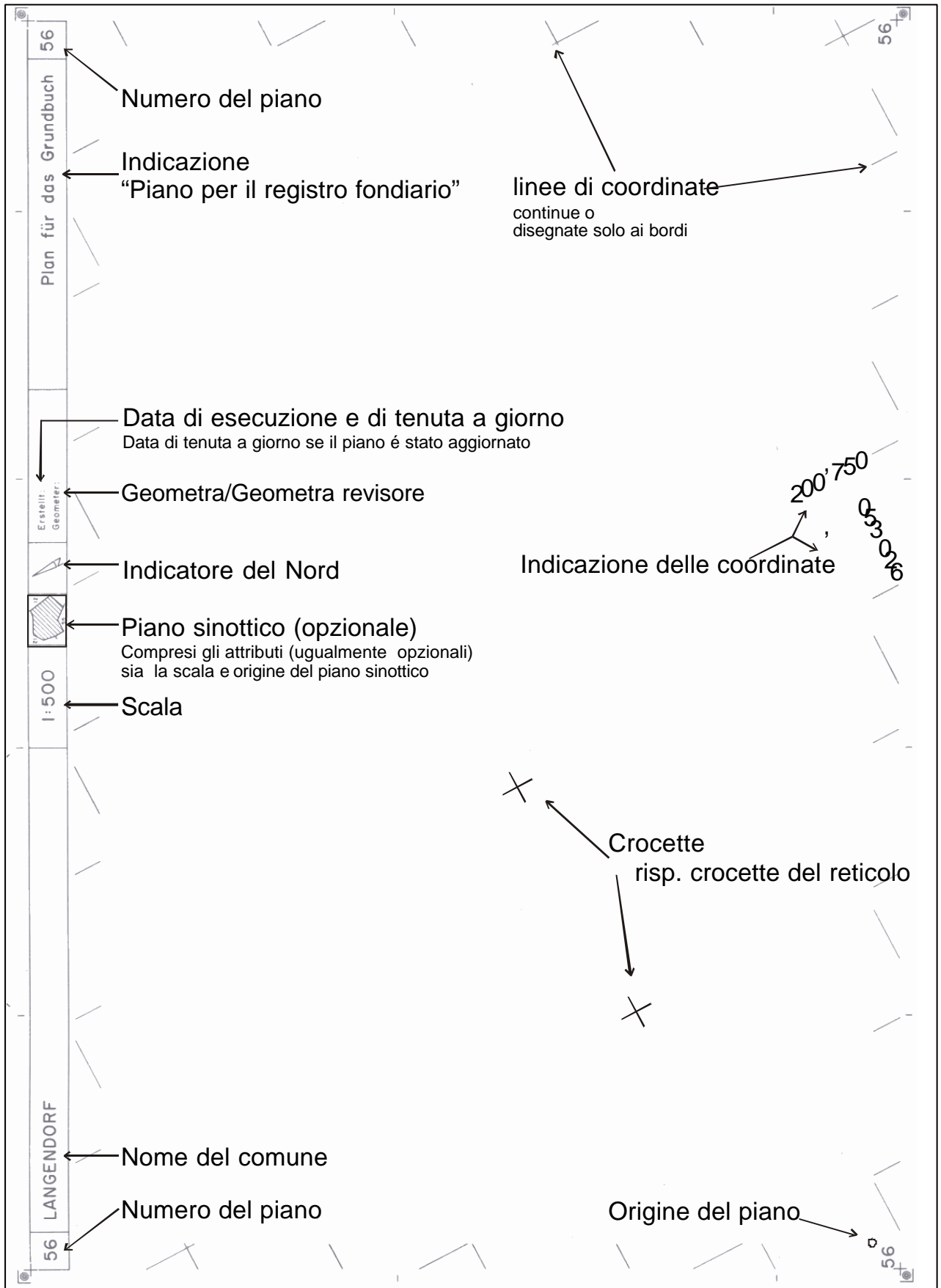
Figura 7: Esempio di piano-quadro e relative spiegazioni.
